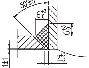
D1,D2,D3,D4 焊接详图 Welding detail of D1,D2,D3,D4 NO SCALE
